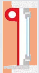
Pose en semi-applique
