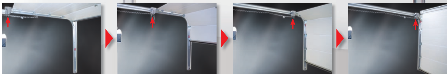
Représentation du mouvement du bloc moteur fixé sur le rail de la porte lors d'une manœuvre de fermeture.
