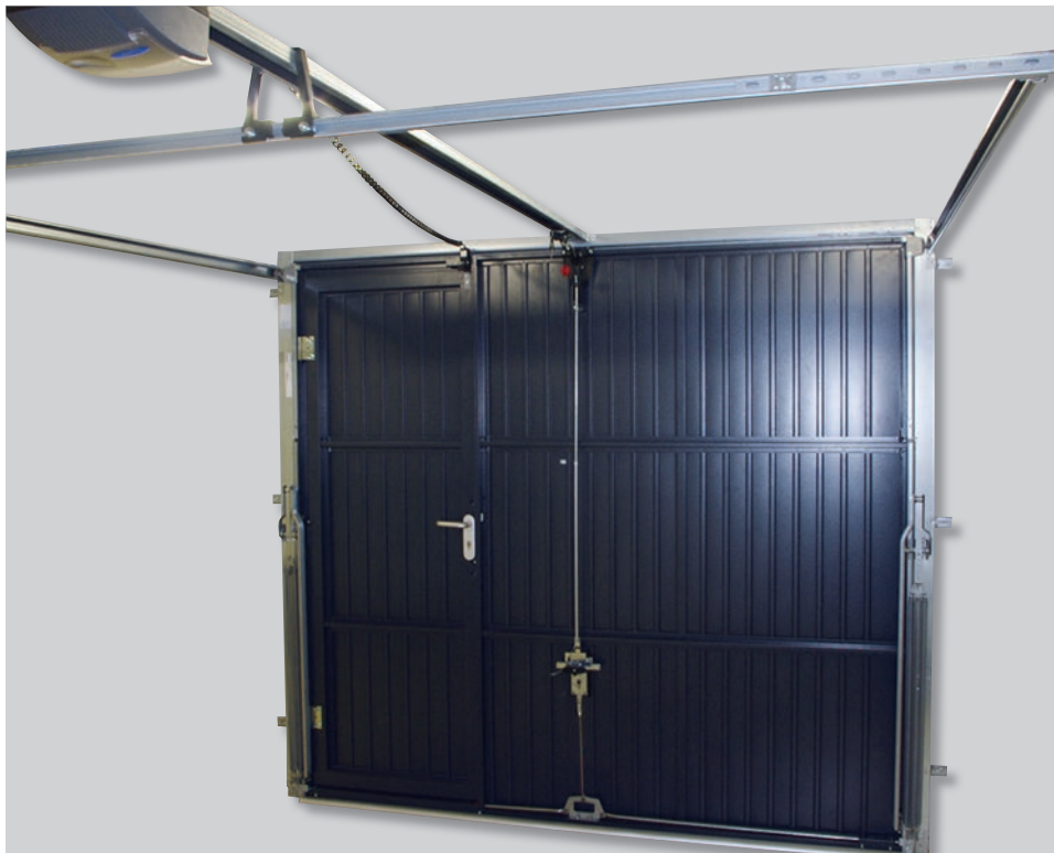
Porte basculante DL avec portillon piéton. Automatisme Integraport® LED. Option : sécurité électrique sur portillon.
